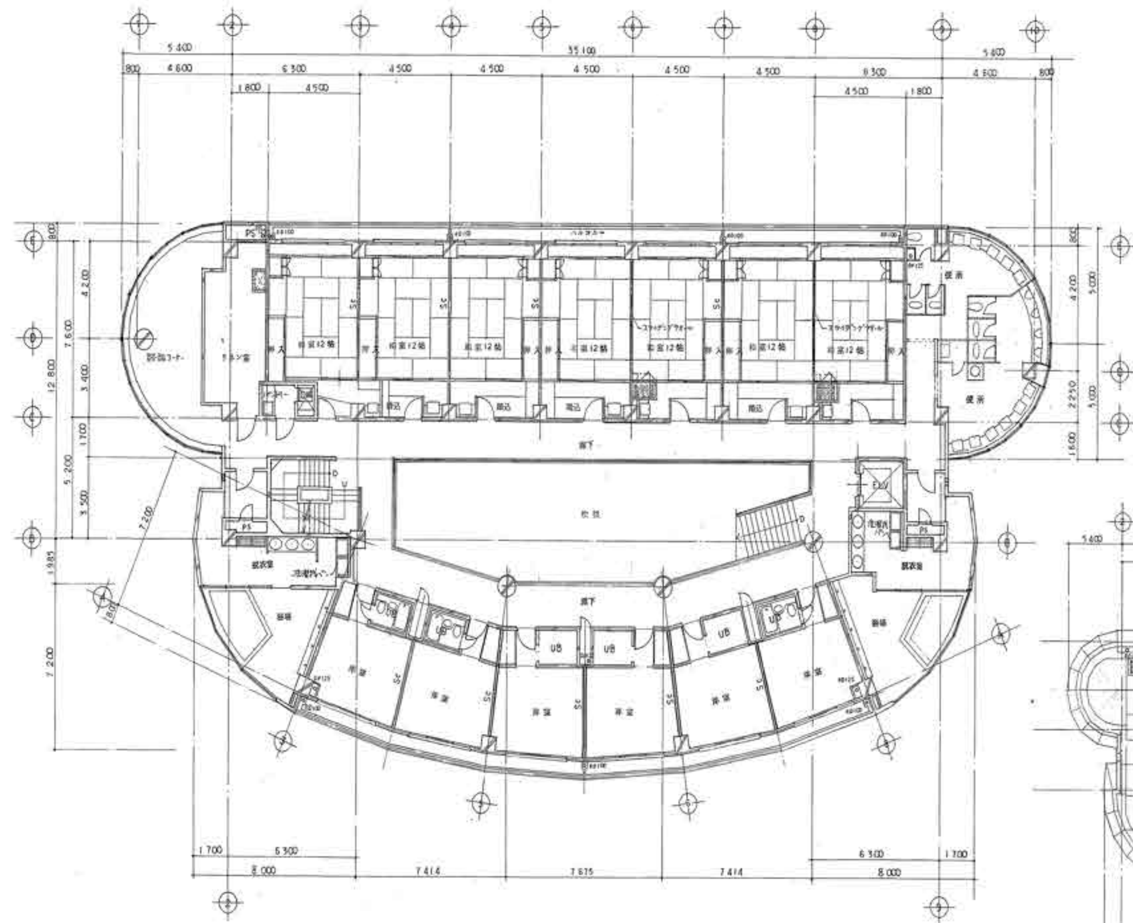
2 樓 平 面 圖 1:100
