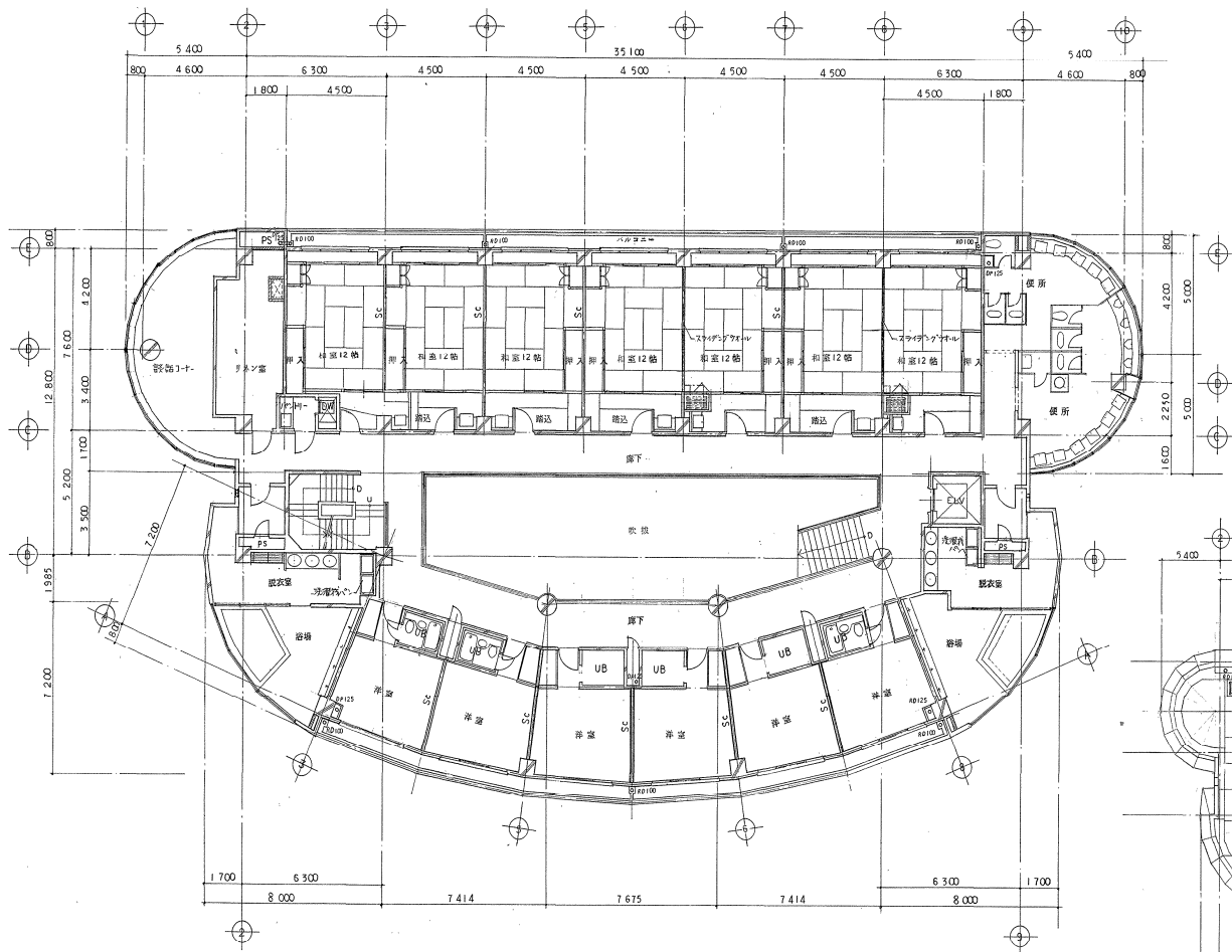
2 階 平 面 図 1:100
