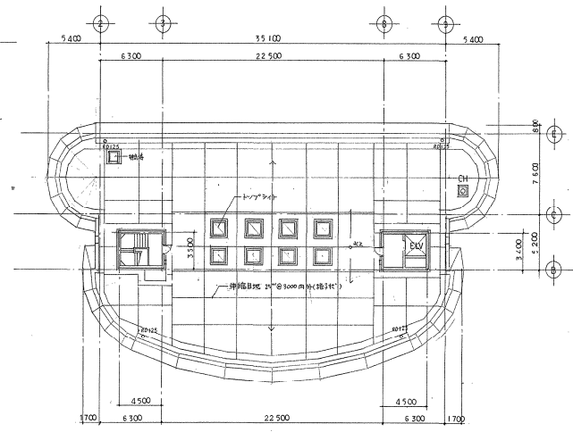
R 階 平 面 図 1:100
