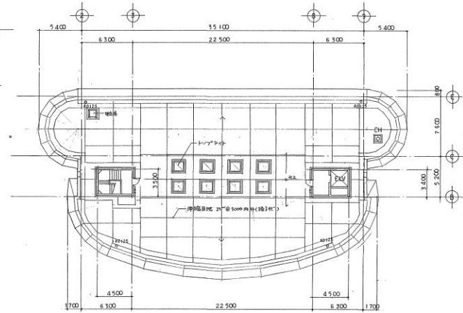
R階平面図 1/100
