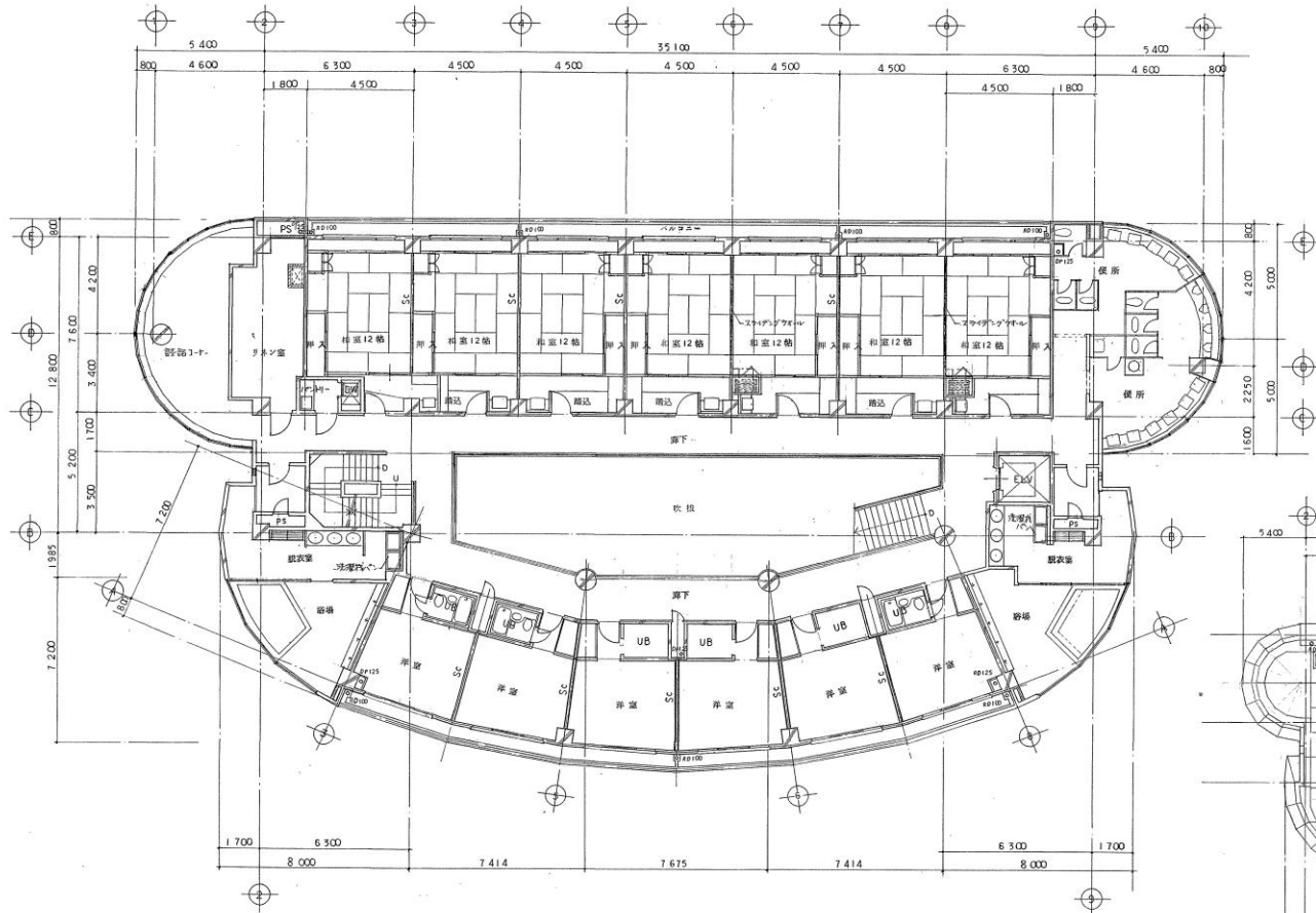
2階平面図 1/100
