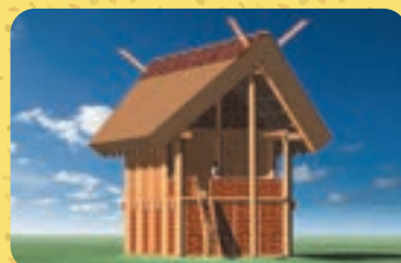
下鉤遺跡 大型建物復元図
